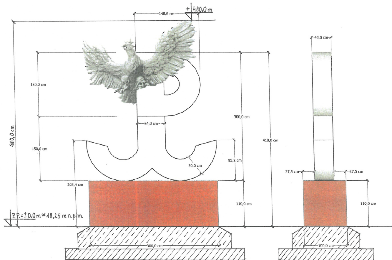
Posadowienie na płycie fundamentowej wg. opracowania branży konstrukcyjnej
