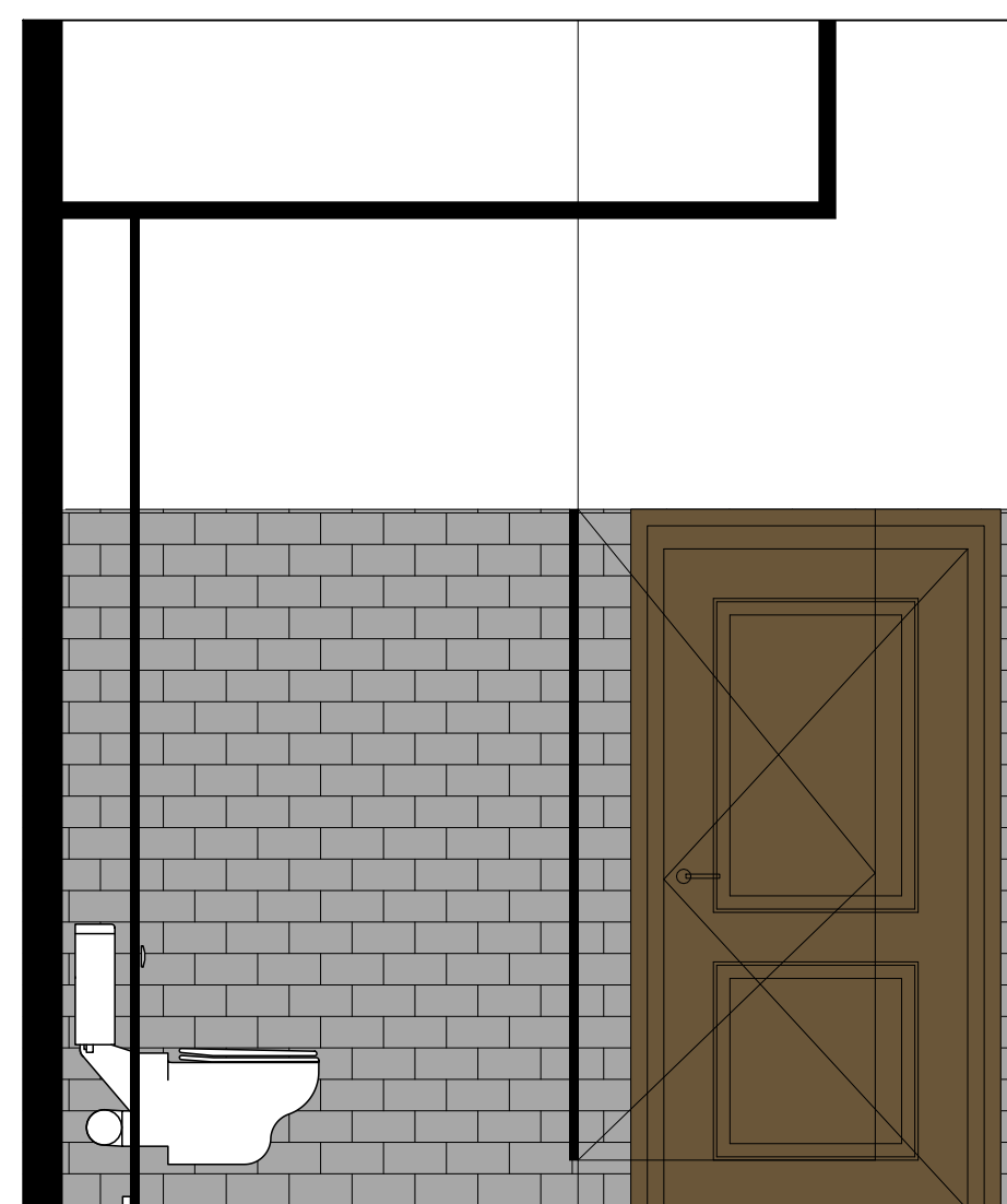
ŚCIANA 8-8
