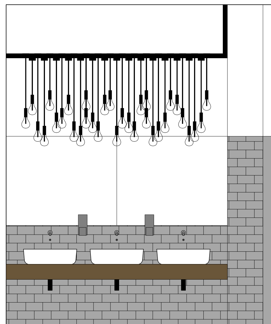
ŚCIANA 2-2
