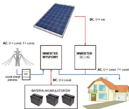
Rysunek 27 Schemat instalacji mieszanej 214 (oznaczenia: DC- prąd stały, AC-prąd przemienny, U- napięcie, f-częstotliwość, var.-zmiennie, const.- stałe)
