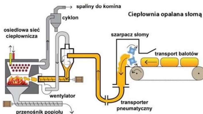
Rysunek 19 Instalacja na pelety 202
