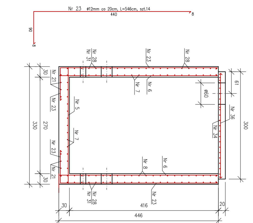
PRZEKROJ B-B
