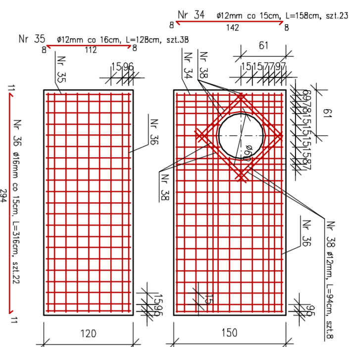
PRZEKROJ B-B
