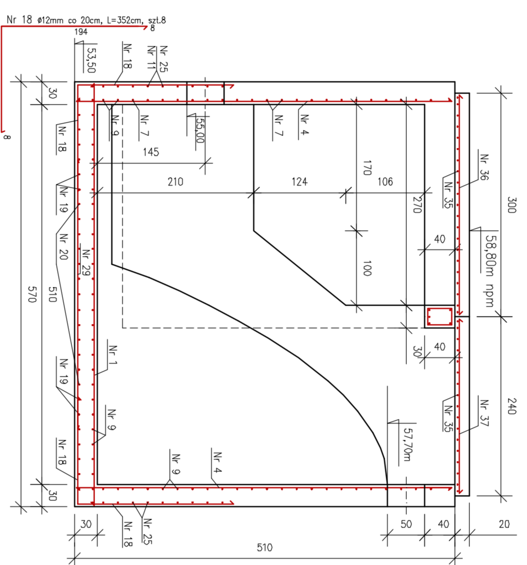
PRZEKROJ A-A
