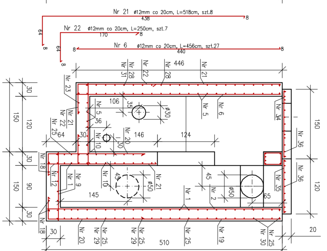
PRZEKROJ C-C
