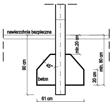
PRZEKRÓJ 1:25
