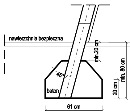
PRZEKRÓJ 1:25
