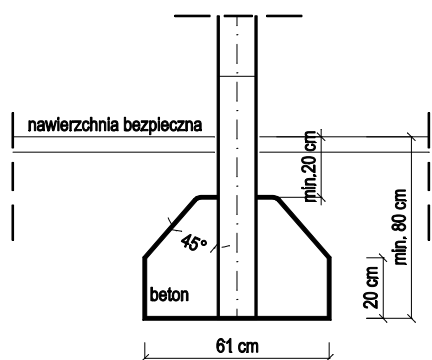
PRZEKRÓJ 1:25
