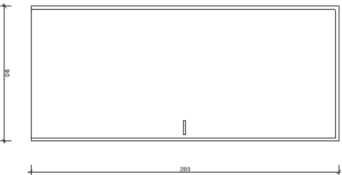
Drzwi lewe, ościeznica drewniana
