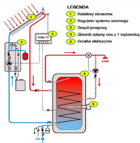
Rysunek 18 Schemat typowej instalacji słonecznej do podgrzewania ciepłej wody użytkowej 198
