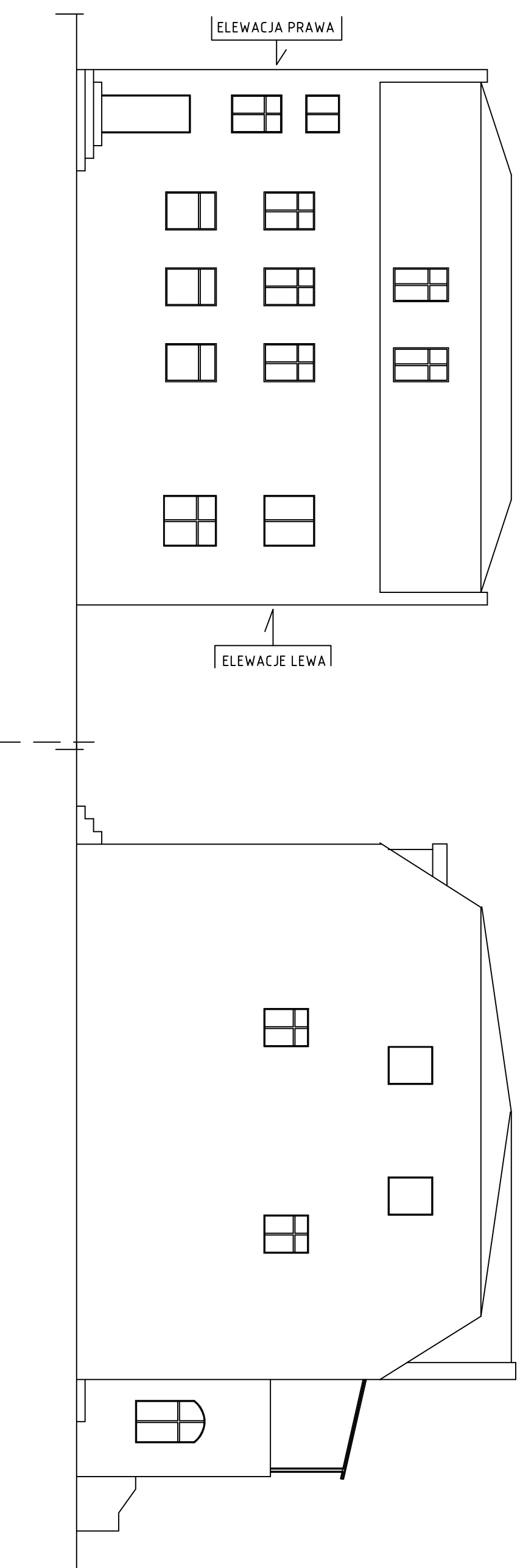
ELEWACJA TYLNA 1 : 100
