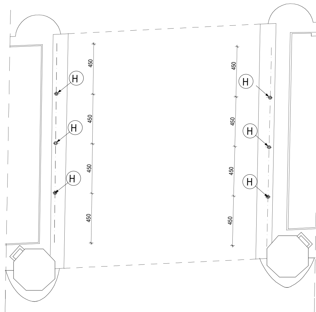
RZUT PRZĘŚLA ŚRODKOWEGO- 1 :200
