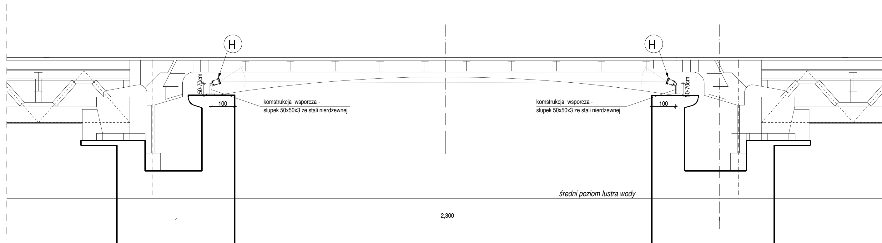
PRZEKRÓJ PRZĘŚLA ŚRODKOWEGO- 1 :100
